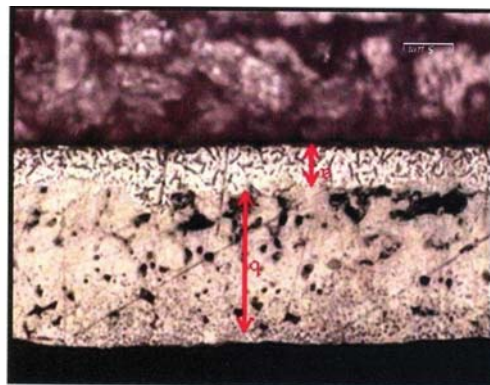
تصویر ۶. بافت متخلخل لایه طلا بزرگ‌نمایی ۱۰۰۰ برابر، منبع: یافته‌های تحقیق
