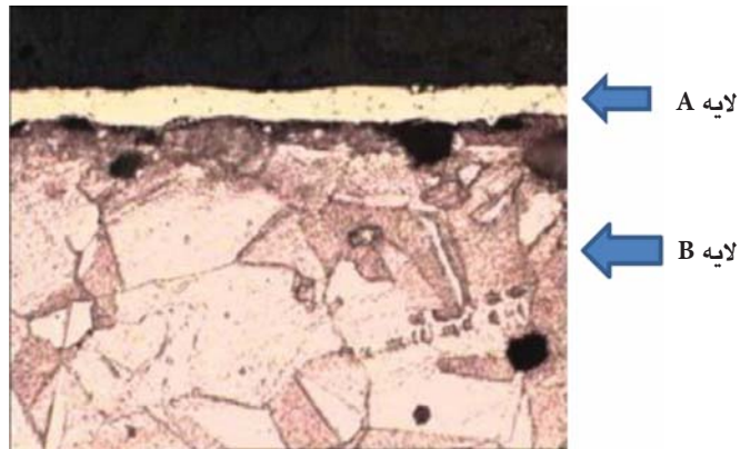
تصویر ۲. عکس میکروسکوپی، نمایش مقطع عرضی لایه‌های طلا و فلز پای. بزرگ‌نمایی X۱۰۰۰، منبع: یافته‌های تحقیق
