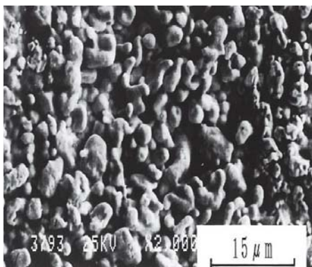
تصویر ۷. بافت متخلخل لایه طلا بزرگ‌نمایی ۲۰۰۰ برابر، تهیه شده با میکروسکوپ روبشی، منبع: یافته‌های تحقیق
