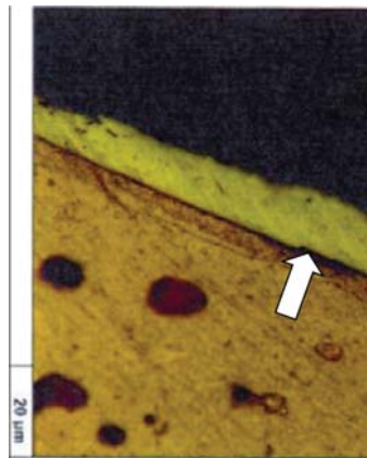
تصویر ۳. عکس میکروسکوپی، نمایش مقطع عرضی نمونه. بزرگ‌نمایی تصویر ۵۰۰ برابر، علامت، محل تشکیل آلیاژ طلا-جیوه و مس را نشان می‌دهد، منبع: یافته‌های تحقیق
