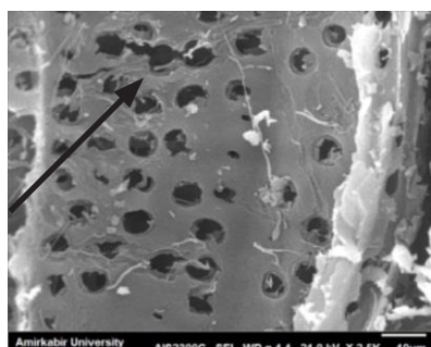
تصویر ۱۱. تصویر SEM از مقطع عرضی نمونه چوب تاریخی چنار با بزرگنمایی m\mu 50 در تصویر سمت راست و نمایش اندازه ریشه‌های قارچ و m\mu 10 در سمت چپ با نمایش اندازه حفرات تخریب شده، منبع: نگارنده اول
