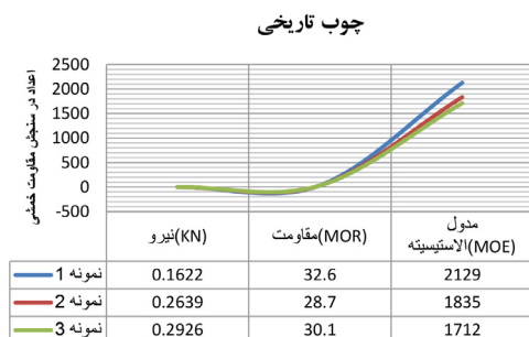
تصویر ۳۱. جدول و نمودار میزان مقاومت خمشی در نمونه‌های چوب چنار تاریخی کلیسای بیت اللحم اصفهان
