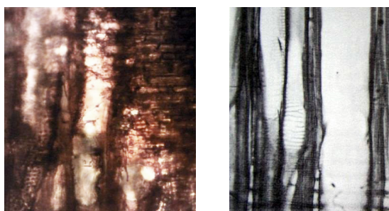
تصویر ۹. سمت راست دیواره آوندی در چوب چنار سالم در برش شعاعی (شواین گروبر و دیگران، ۱۳۹۰، ص ۱۰۶)، سمت چپ دیواره های آوندی در نمونه چوب سرداب محراب کلیسا از مقطع شعاعی، منبع: نگارنده اول
