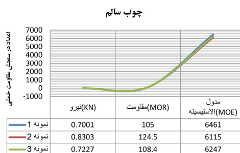
تصویر ۳۰. جدول و نمودار میزان مقاومت خمشی برای نمونه‌های چوب چنار سالم
