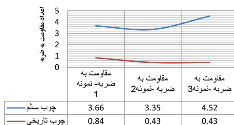
تصویر ۳۹. جدول و نمودار میزان مقاومت ضربه ای نمونه‌های چوب چنار سالم در مقایسه با نمونه‌های چوب تاریخی کلیسای بیت اللحم اصفهان
