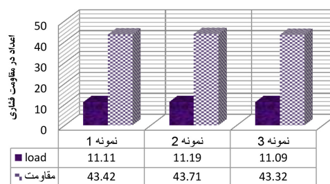
تصویر ۳۵. جدول و نمودار میزان مقاومت فشاری نمونه های چوب چنار سالم
