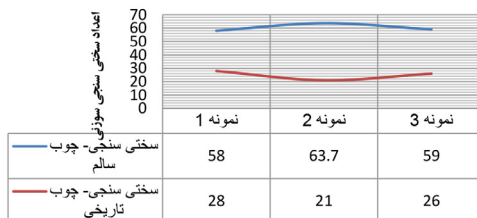
تصویر ۴۵. جدول و نمودار محاسبه سختی سنجی سوزنی در نمونه چوب چنار سالم با نمونه چوب تاریخی کلیسای بیت اللحم اصفهان
