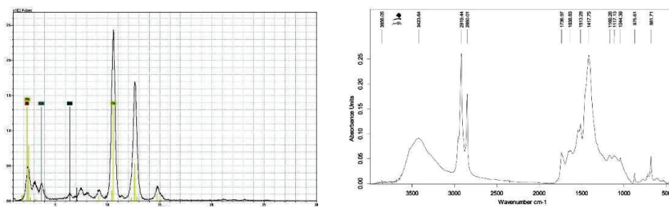
تصویر ۴. (راست): نمودار FTIR مربوط به نمونه W1. (چپ): نمودار XRF مربوط به نمونه W1. در جدول شماره ۲، پیک‌های دو نمونه سفید و مقایسه آنها با پیک‌های شاهد مشاهده می‌شود. منبع: نگارنده
