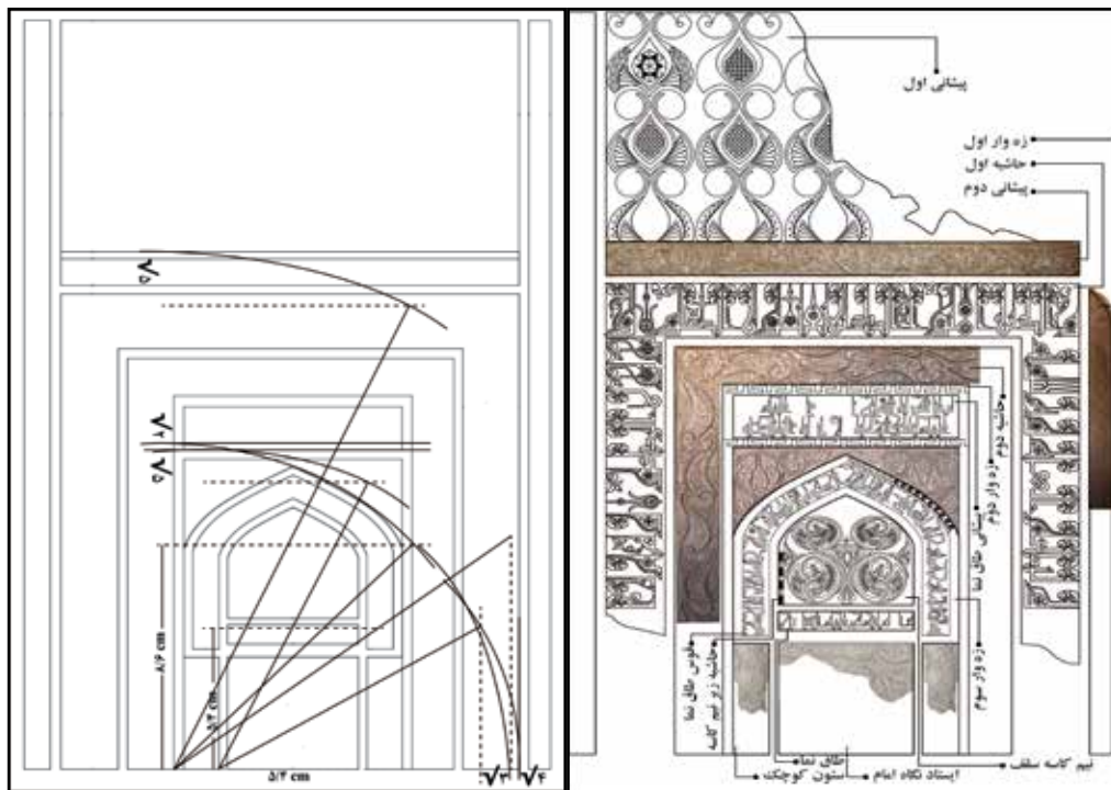
تصویر ۱۲-تناسبات طلایی مربع شاخص ۵ و ۴ و ۸ و ۱۰ سانتی متر مسجد مدرسه زوزن با مقیاس تقریبی ۱۰/۶ برابر کوچک شده است (مأخذ: نگارنده)
