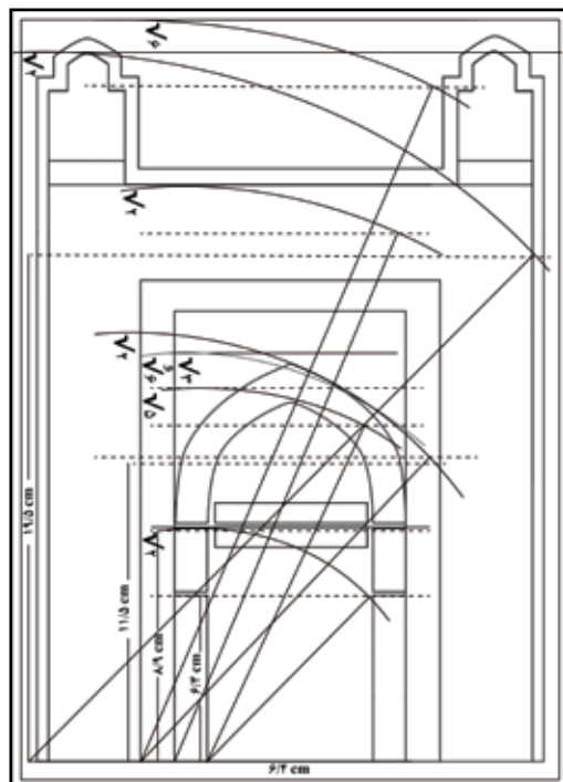
تصویر ۲۵- تناسب طلایی مربع شاخص ۴ و ۶، ۹ و ۱۱ و ۱۹ سانتی متر مسجد فرومد با مقیاس تقریبی ۱/۶ برابر کوچک شده است (مأخذ: نگارنده)
