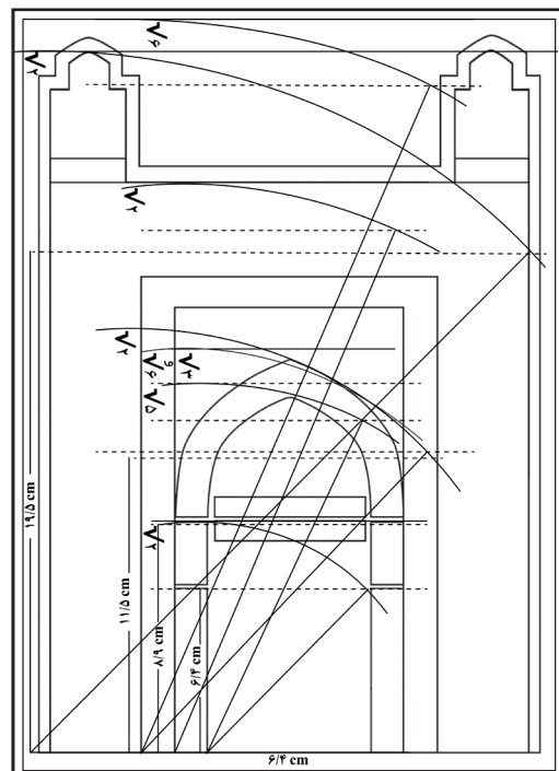
تصویر ۲۵-تناسبات طلایی مربع شاخص ۴و۶، ۹و۸، ۱۱و۵ و ۱۹۵ سانتی متر مسجد فرومد با مقیاس تقریبی ۱۰/۶ برابر کوچک شده است (مأخذ: نگارنده)
