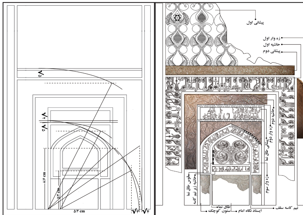
تصویر ۱۲- تناسبات طلایی مربع شاخص ۵۰۴ و ۸۰۶ سانتی متر مسجد مدرسه زوزن با مقیاس تقریبی ۱۰/۶ برابر کوچک شده است (مأخذ: نگارنده)
