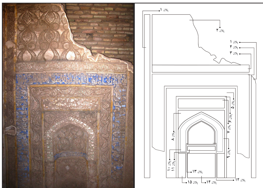
تصویر ۳- تصویر پلان بندی محراب مسجد-مدرسه زوزن (مأخذ: نگارنده)
